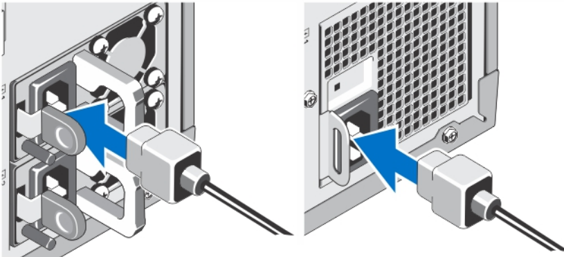
그림 3. 전원 케이블 연결
