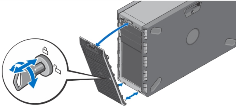
그림 6. 베젤 설치
